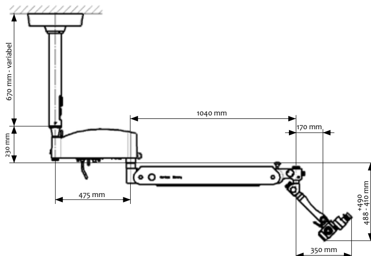
SOM® 62 - Rollstativ
