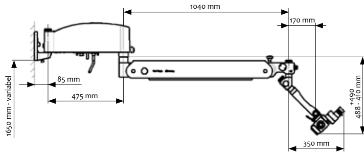
SOM® 32 - Deckenmontage
